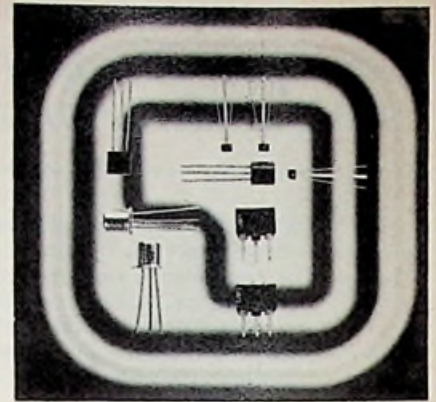
Afb. 4. Epitaxiale PNP siliciumplanair transistor voor LF voorversterker- en drivertrappen. De afmetingen van het kristalplaatje zijn 0,5 x 0,5 mm.
